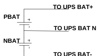
Diagrama de cableado de bloques Terminal para 30K/40K
