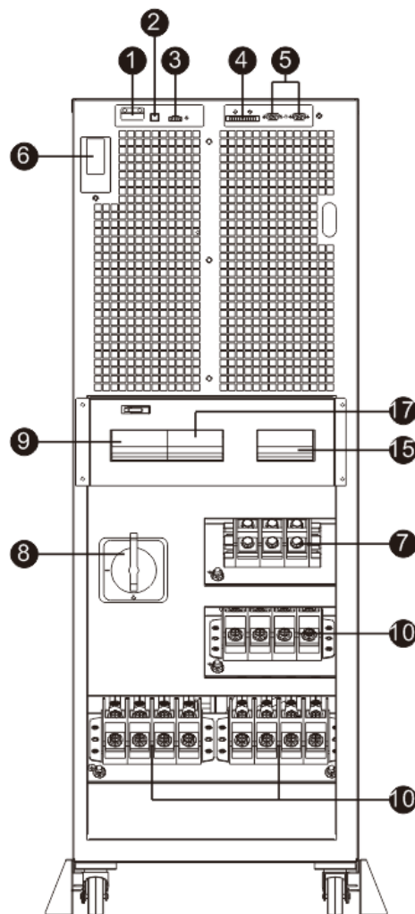
Diagrama 4: 40K aVista frontal con puerta abierta
