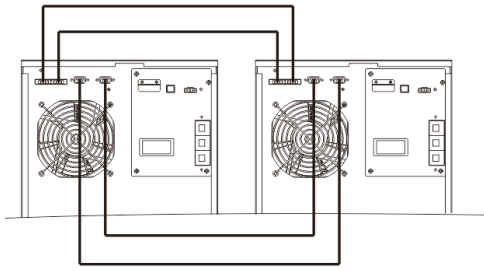
Diagrama 1: Dos SAI en paralelo
